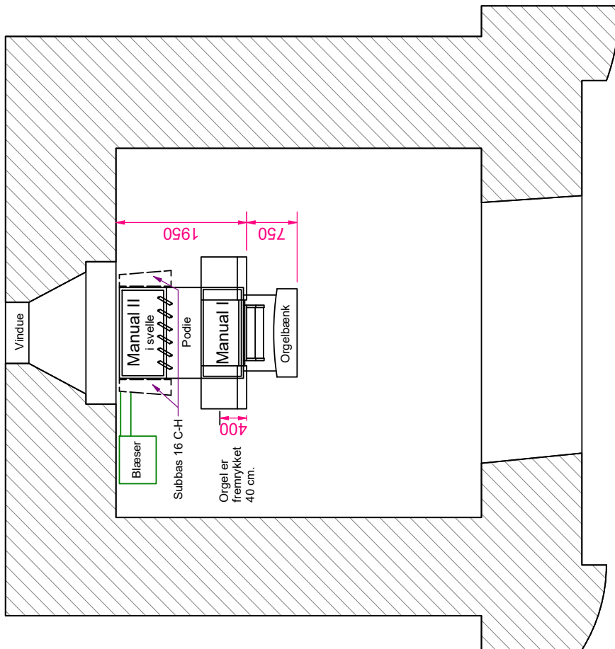
Plan ( 1 : 50 )
