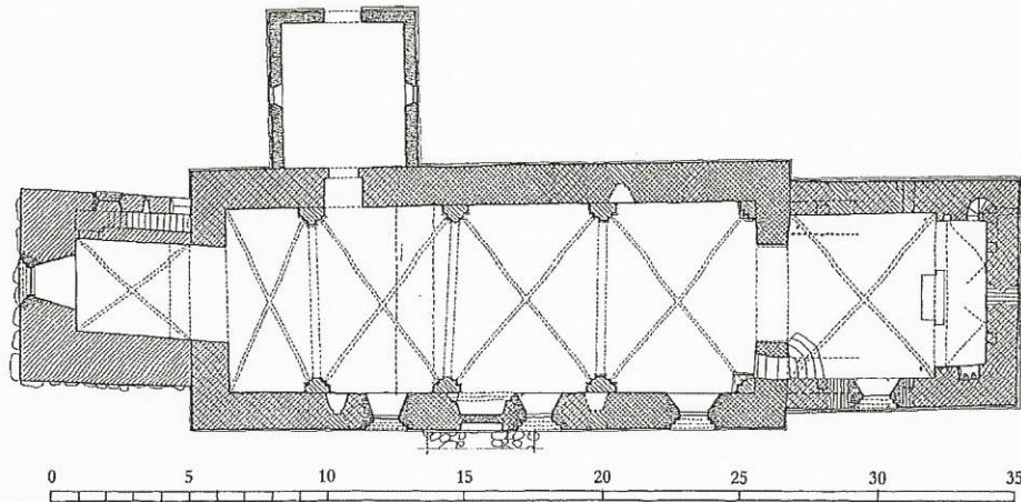
Fig. 5. Sydfacade og plan 1:300. Målt af Rolf Graae 1941 og Vilhelmsen, Marxen og Bech-Jensen 1991, tegnet af henholdsvis Rolf Graae 1941 og KdeFL 1996. – South elevation and ground-plan.
